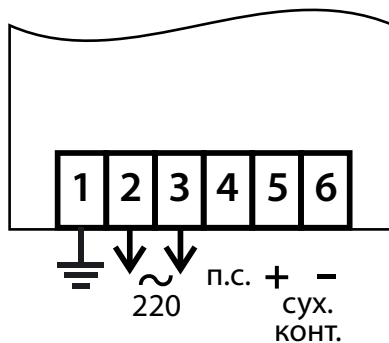
Рис. 1. Схема подключения LCL24PM/12P
