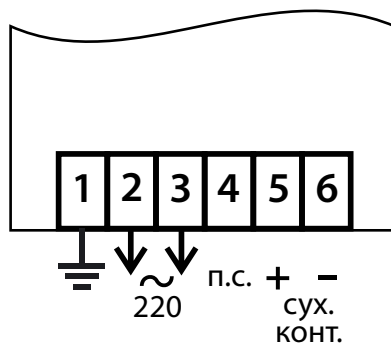
Рис. 1. Схема подключения LCL24PM/24P
