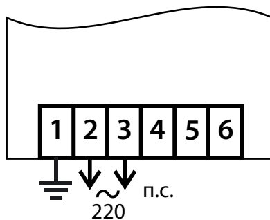
Рис. 1. Схема подключения LCL40PP/40S1
