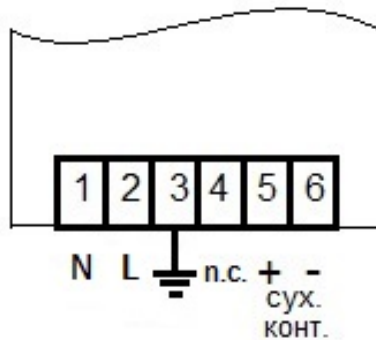
Рис. 1. Схема подключения LCL24PM/12P
