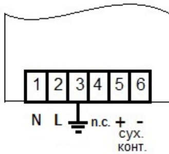
Рис. 1. Схема подключения LCL24PM/24M
