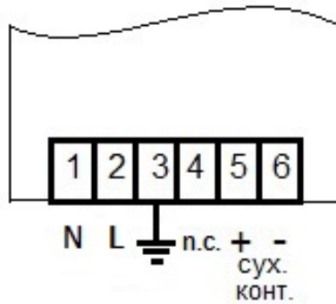
Рис. 1. Схема подключения LCL24PM/24P
