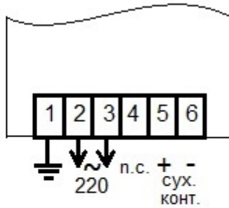
Рис. 1. Схема подключения LCL24PM/36M
