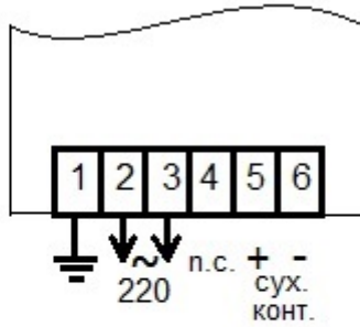
Рис. 1. Схема подключения LCL40PP/1-G
