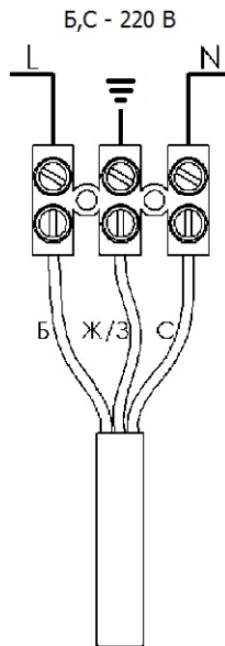
Рис. 1. Схема подключения LCL40PP/120S
