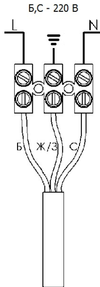
Рис. 1. Схема подключения LCL40PP/160S
